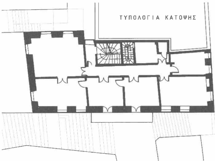
Σχ. 2. Τυπολογία κάτοψης. Κεντρικός διάδρομος σε προσανατολισμό Β-Ν που τροφοδοτεί τους χώρους εκατέρωθεν. Κλιμακοστάσιο και βοηθητική σκάλα στην ανατολική πλευρά.
