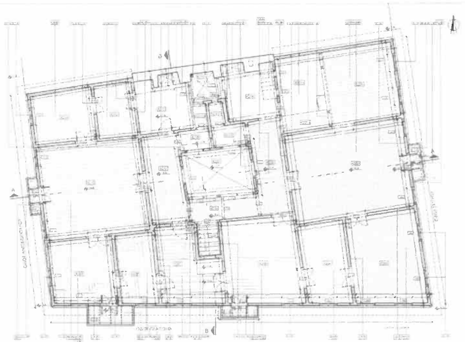
Εικ. 11. Κτίριο Αρμανσπεργκ – κάτοψη β' ορόφου.
