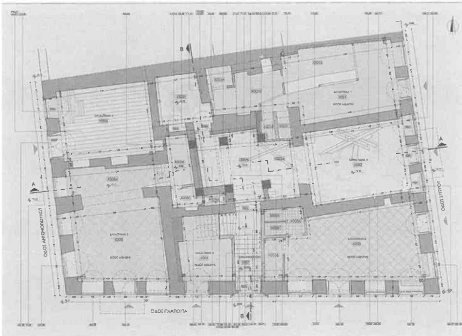
Εικ. 2. Κτίριο Άρμανσπεργκ: Κάτοψη στάθμης ισόγειου – αποτύπωση.
