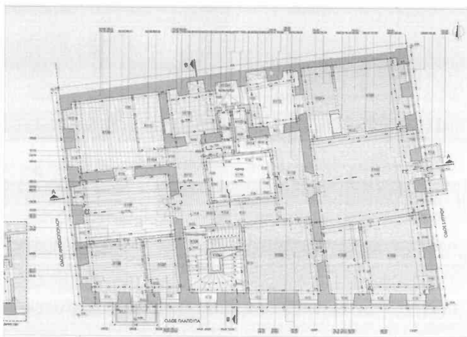
Εικ. 8. Κτίριο Αρμανσπεργκ – κάτοψη α΄ ορόφου – αποτύπωση.
