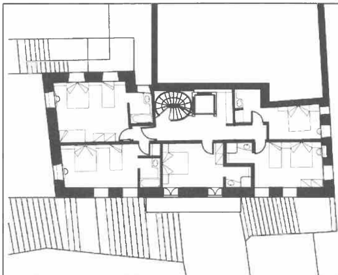
Σχ. 4. Κάτοψη πρότασης αποκατάστασης.
